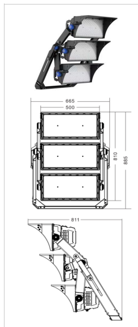
SL-01C-1500W
