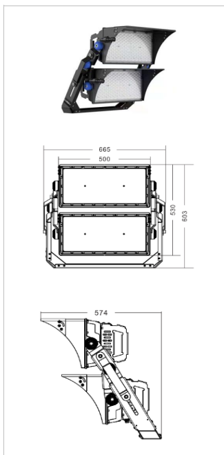
SL-01B-1000W
